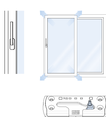
Безопасная, энергосберегающая вентиляция (зазор до 6 мм по всему периметру створки)
