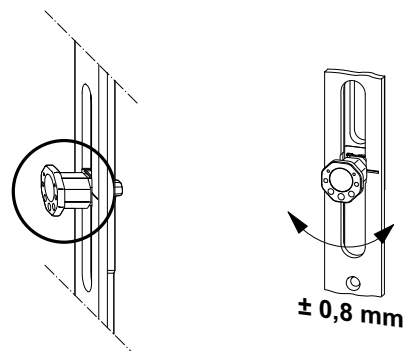
Регулировка усилителей
