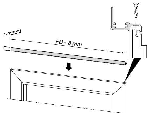
Направляющая створки
