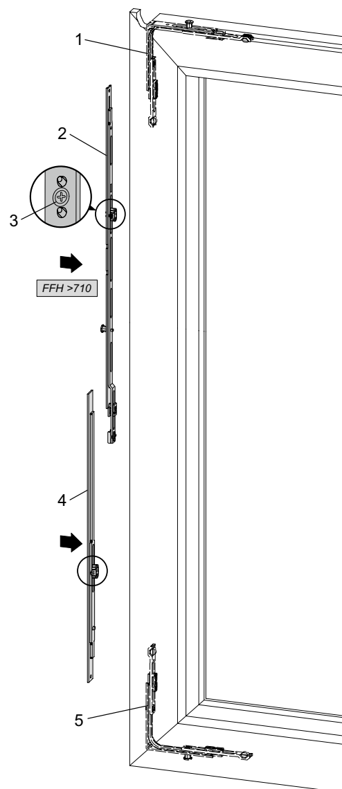
Блокада с соединителем (устанавливается вертикально)
