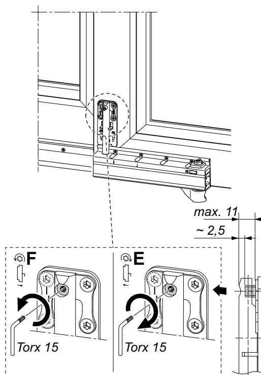
Регулировка усилителей
