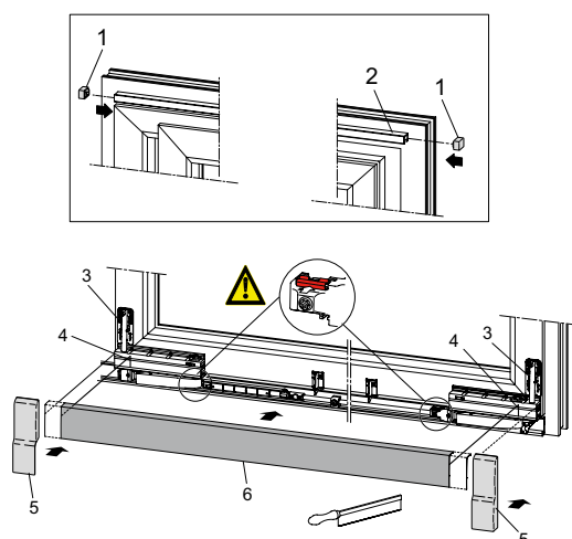
Нижние накладки
