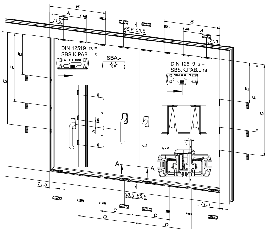
Позиции ответных планок в штапеловых окнах – 2 створки раздвижные (штапеловое окно)
