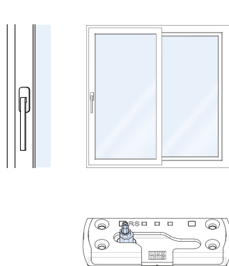
Положение „закрыто”
