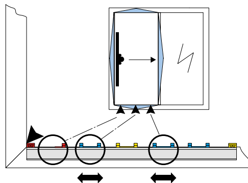
SBS.K.PAB... и SBA.K... устанавливаются горизонтально (внизу)
