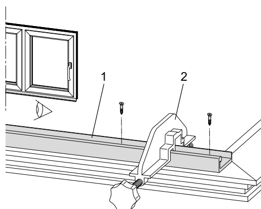
Шаблон для монтажа нижней направляющей на раму
