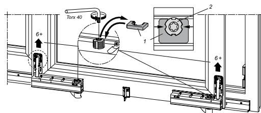
Регулировка створки
