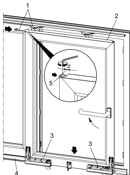
Установка створки на раму
