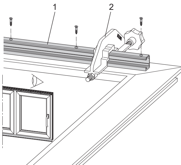
Шаблон для монтажа верхней направляющей на раму
