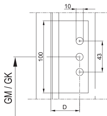
Сверление и фрезеровка отверстий GAK/ GAM ...D 25 ...50 - D = межосевое расстояние замка
