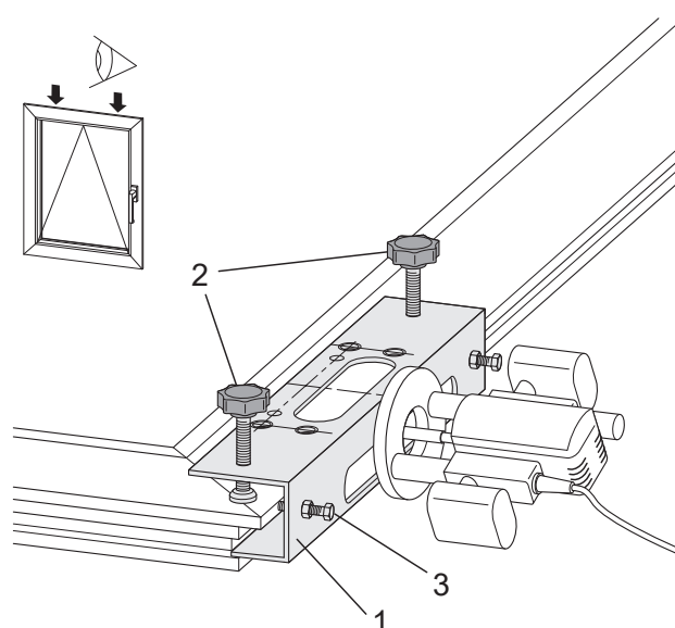
Фрезерование под верхнюю шину в угловой части створки
