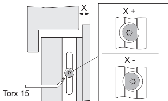
Эксцентрические ролики
