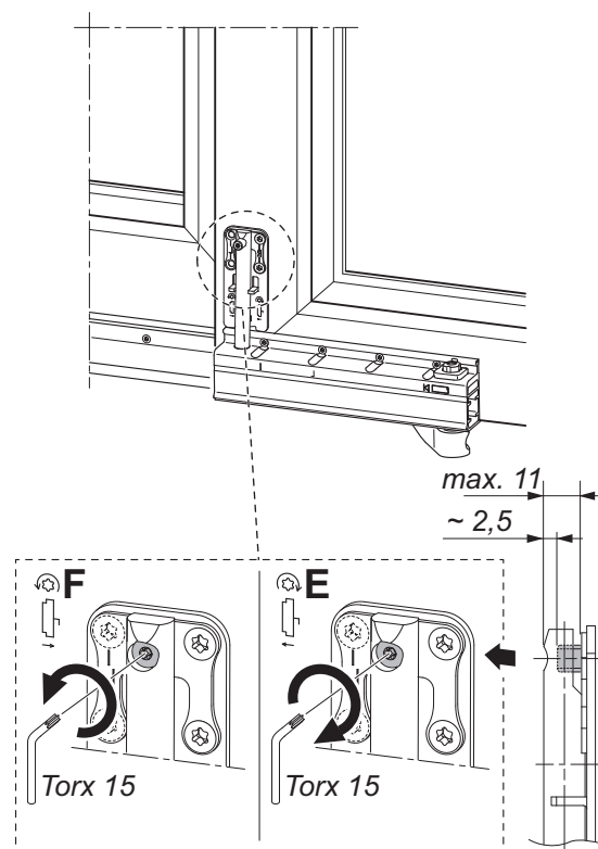
Регулировка усилителей
