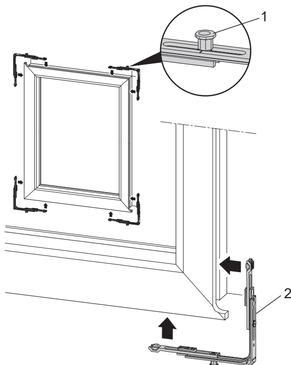
Угловые передачи
