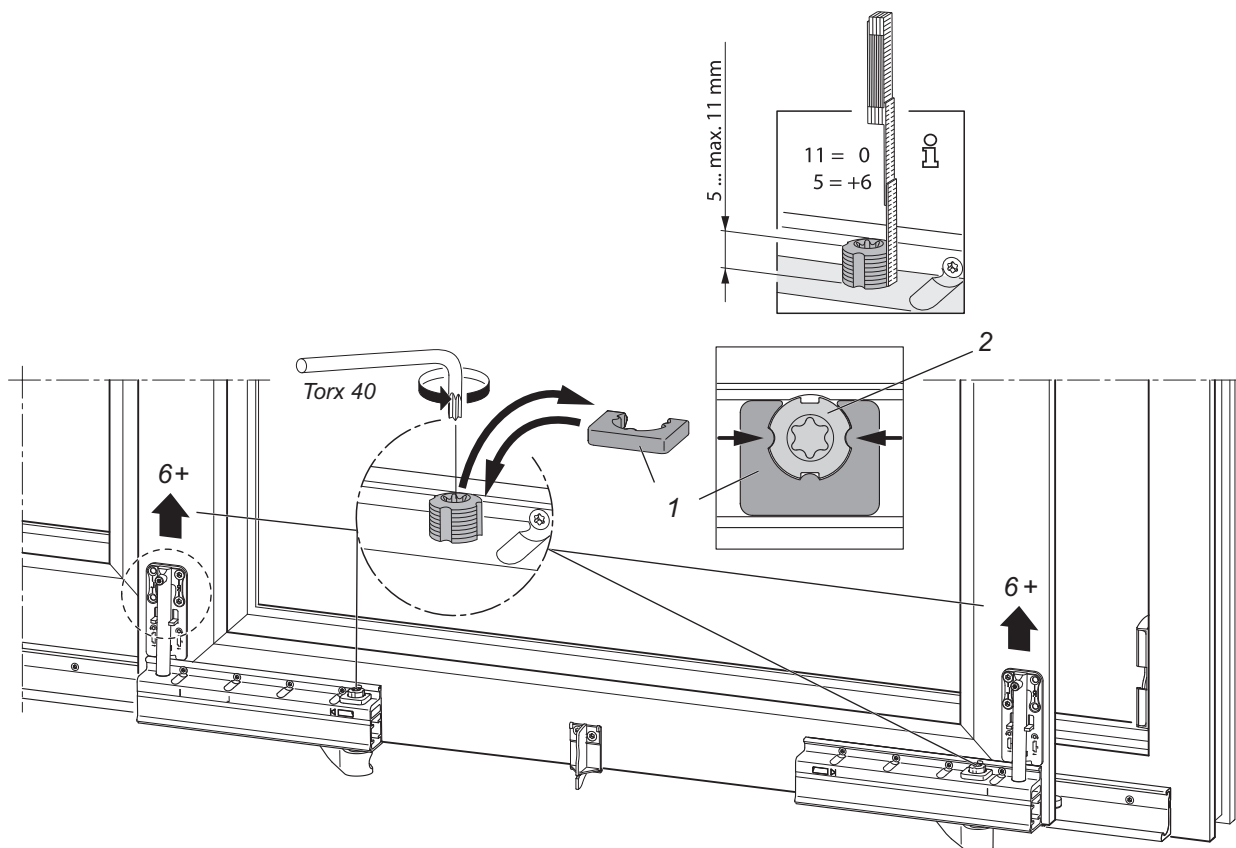
Регулировка створки
