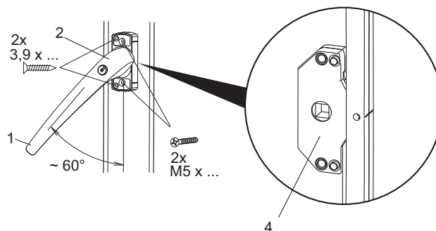
Засов с шестеренчатой передачей движения
