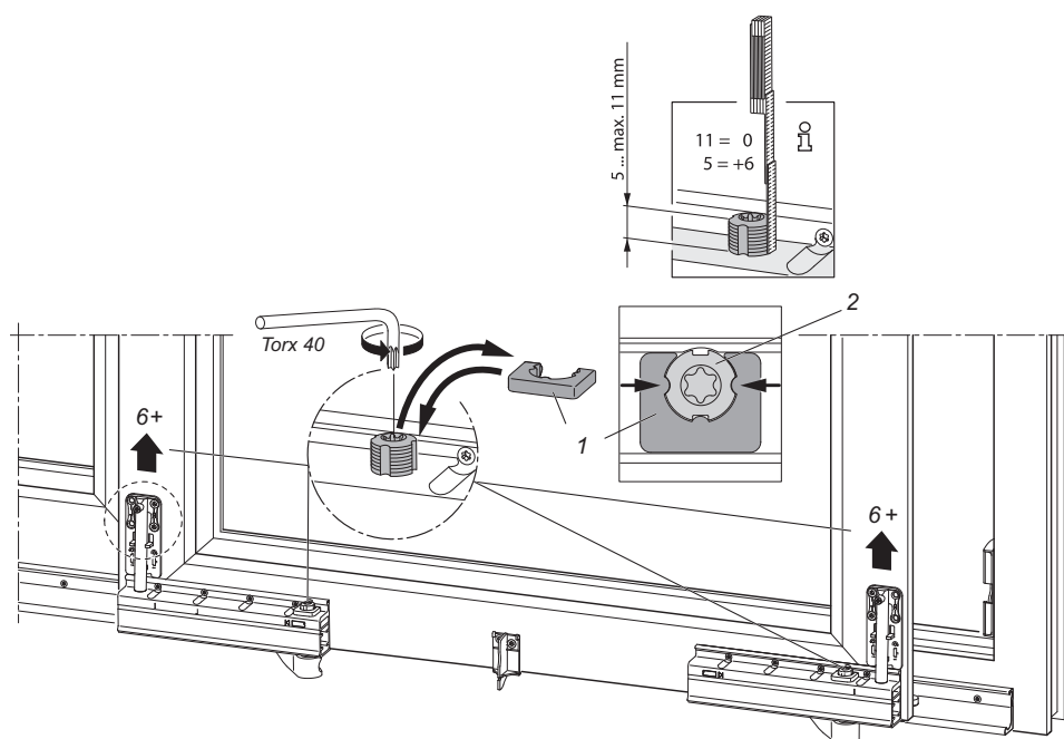
Регулировка створки
