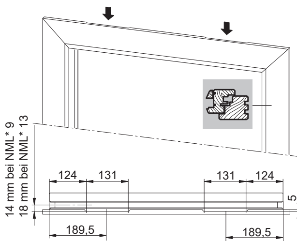
Фрезерование в верхнем нахлесте * NML = Nutmittenlage (расстояние от оси фурнитурного паза до края рамы)
