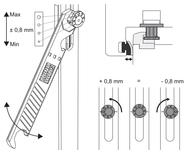
8-гранная цапфа
