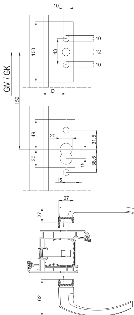
Сверление и фрезеровка отверстий GAKA/ GAMA D ... - D = межосевое расстояние замка
