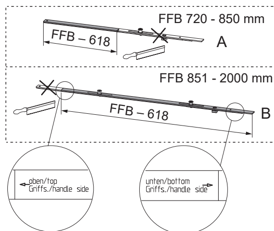
Соединительная шина (нижняя/ устанавливаемая горизонтально)
