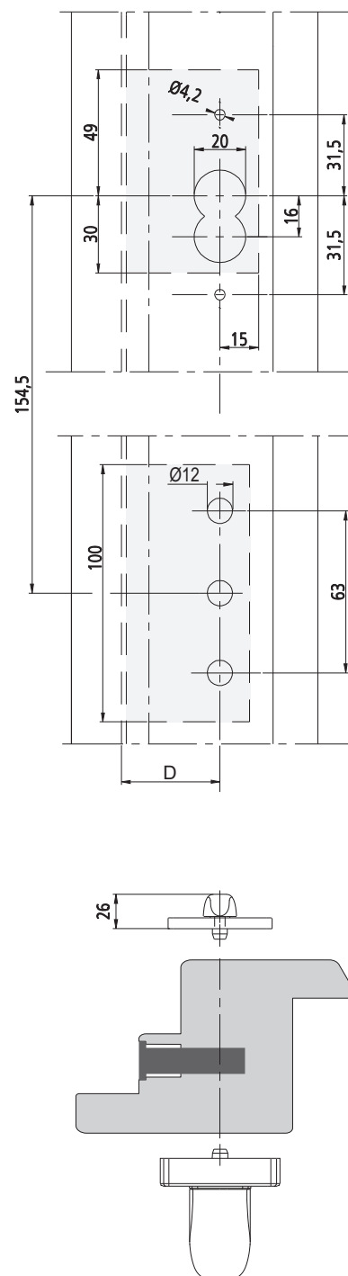
Чертежи монтажных отверстий под засов SK-A D = межосевое расстояние замка
