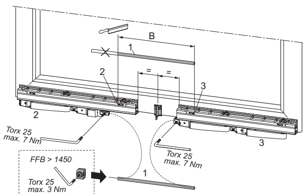
Соединительный прут
