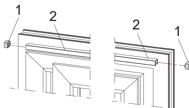
Заглушки направляющей
