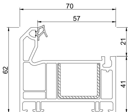
Рама 62 мм
