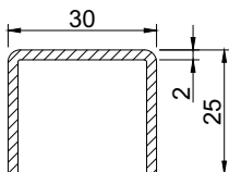
Усилитель Арт. № S793715 I_g=1,5 \text{ см}^4 I_w=1,9 \text{ см}^4
