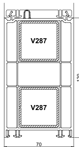
Расширитель 120 мм Арт. № 363
