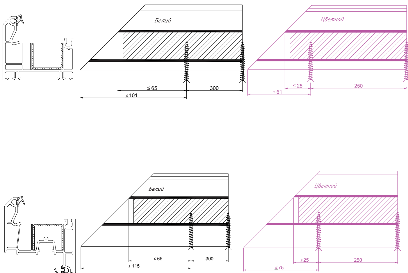
Рис. 2 Крепление вкладышей
