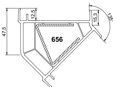
Соединитель угловой 135° Арт. № 6356
