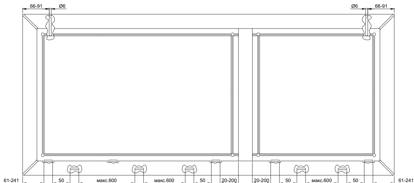
Рис.13 Оконная рама.
