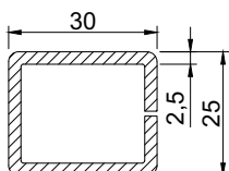
Усилитель Арт. № S93725 I_g=2,2 \text{ см}^4 I_w=2,9 \text{ см}^4
