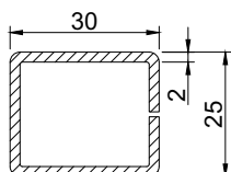
Усилитель Арт. № S793720 I_g=1,8 \text{ см}^4 I_w=2,4 \text{ см}^4
