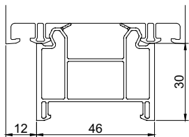
Профиль подставочный 30 мм Арт. № 342
