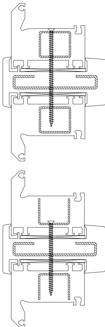
Рис. 7 Примеры соединений
