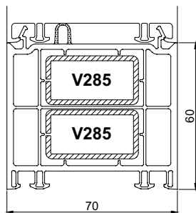
Расширитель 60 мм Арт. № 362
