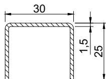
Усилитель Арт. № S791715 I_g=0,7 \text{ см}^4 I_w=1,8 \text{ см}^4
