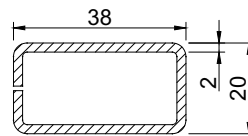
Усилитель Арт. № V285 (604) I_{gv}=1,3 \text{ см}^4 I_w=3,6 \text{ см}^4
