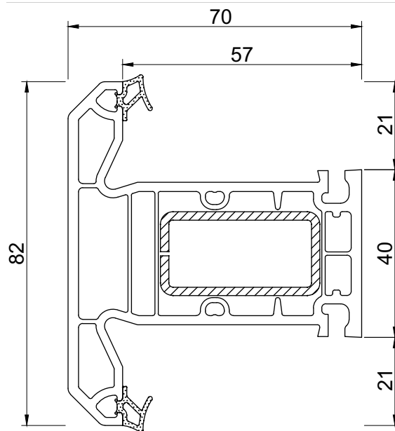
Импост 82 мм
