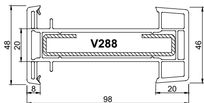
Соединитель H-образный Арт. № 70602 (352)
