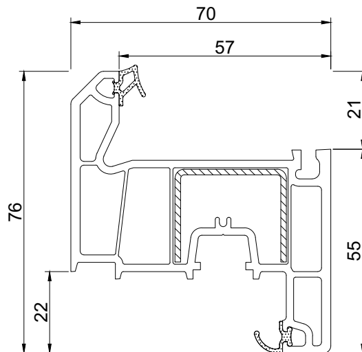
Створка 76 мм
