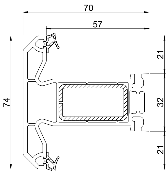
Импост 74 мм
