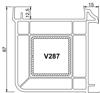
Соединитель угловой 90° Арт. № 70603 (355)
