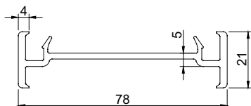
Соединитель балконный Арт. № 70601 (350)
