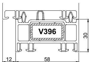
Расширитель 30 мм Арт. № 144
