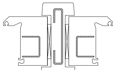
Рис. 2 Соединение с помощью соединителя
