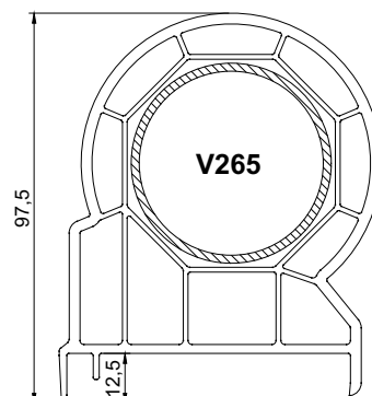
Соединитель угловой Арт. № 70604 (340)
