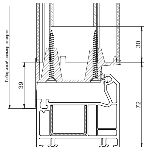
Размер раскроя армирования
