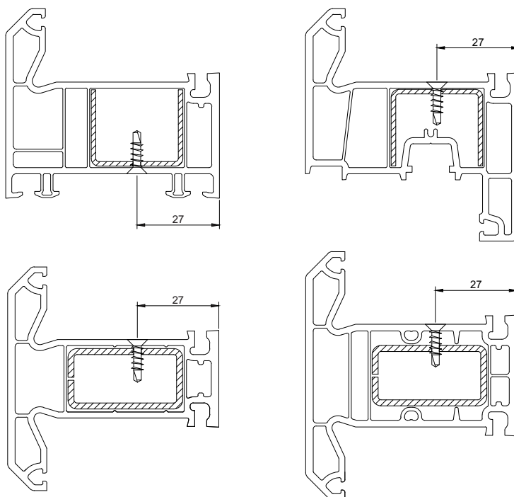
Рис. 3 Ось крепления
