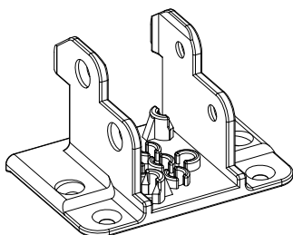
Соединитель импоста Арт. № J043 только для арт.7392
