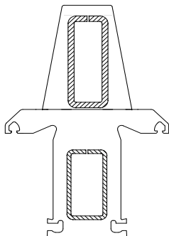
Рис. 3 Применение пилястра
