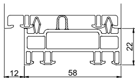
Профиль подставочный 22 мм Арт. № 741
