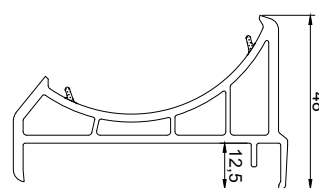
Адаптер к арт. 70604 Арт. № 70605 (341) Монтажный анкер Арт. № S099
