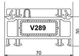
Расширитель 30 мм Арт. № 360
